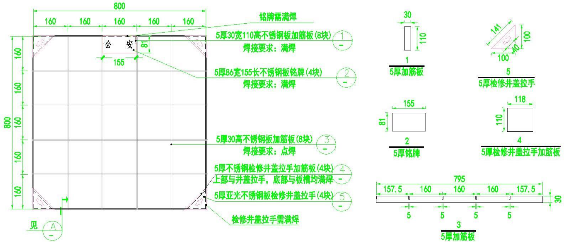
800x800方形公安下沉式井盖详图(尺寸单位均为mm)
