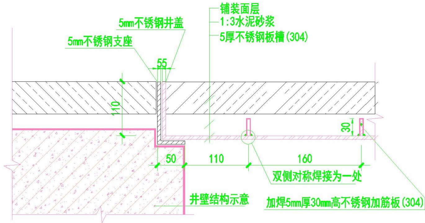
A 铺装上井盖断面详图(尺寸单位均为mm)
