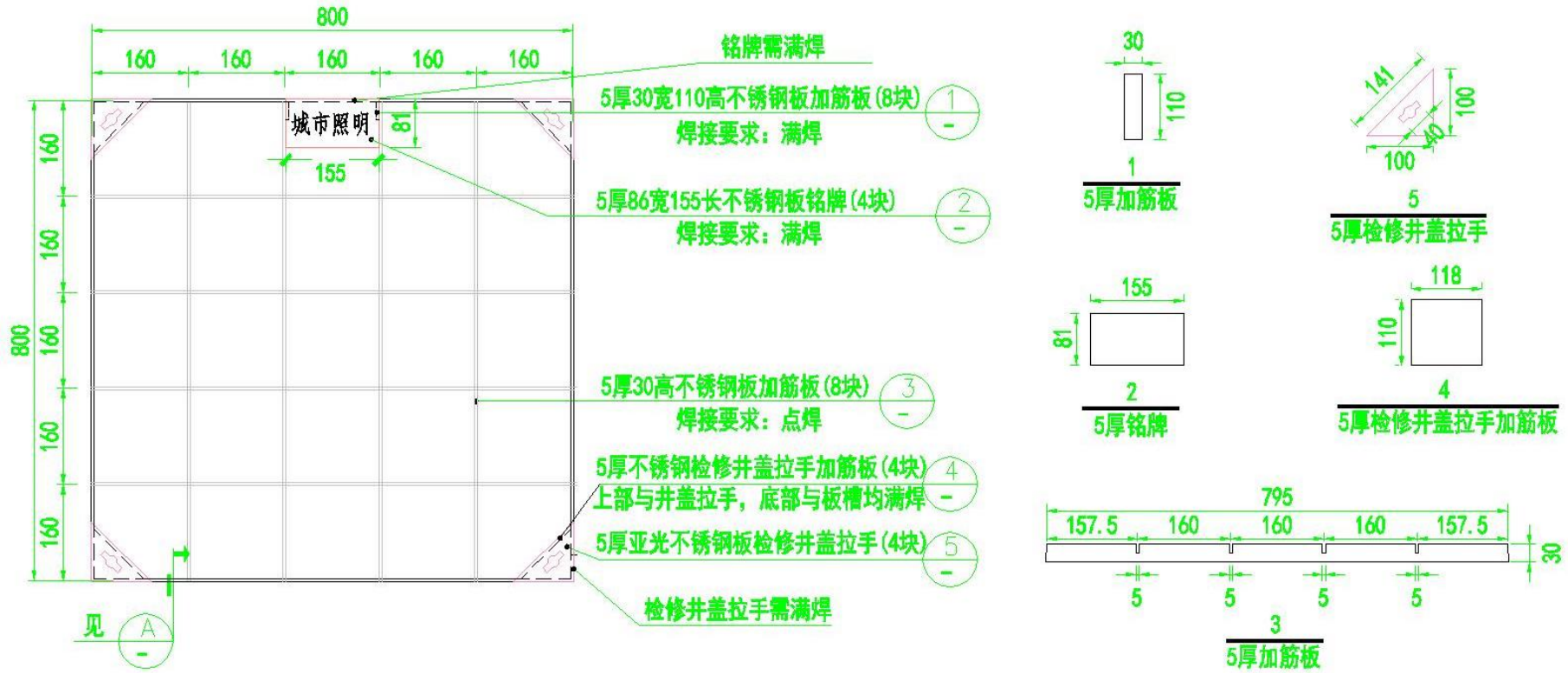
800x800方形路灯下沉式井盖详图 (尺寸单位均为mm)
