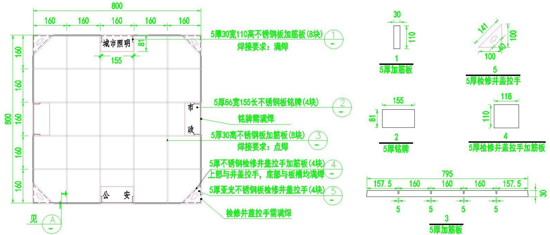
800x800方形多功能下沉式井盖详图(尺寸单位均为mm)
