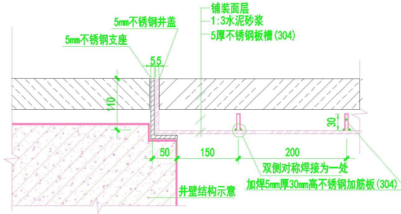
B 铺装上井盖断面详图(尺寸单位均为mm)
