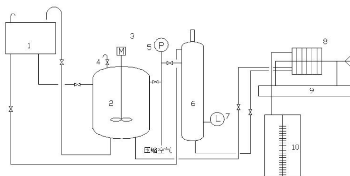
图 1 过滤装置流程图
