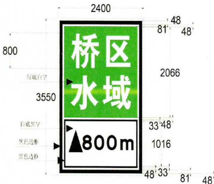
B 型（适合 V 级及以下航道），尺寸单位：mm
