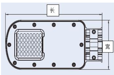
LED 路灯灯头外形尺寸示意 LED 投光灯灯头外形尺寸示意
