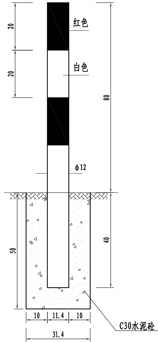
道口标柱
