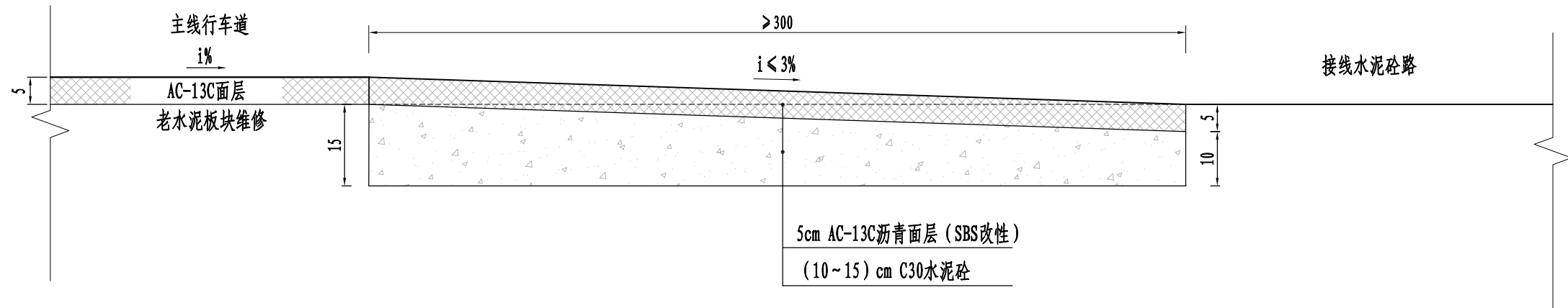
接线工程设计图 (一)
