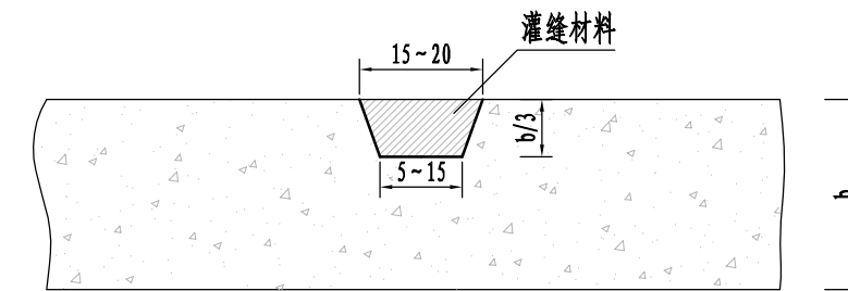
条带补缝法
