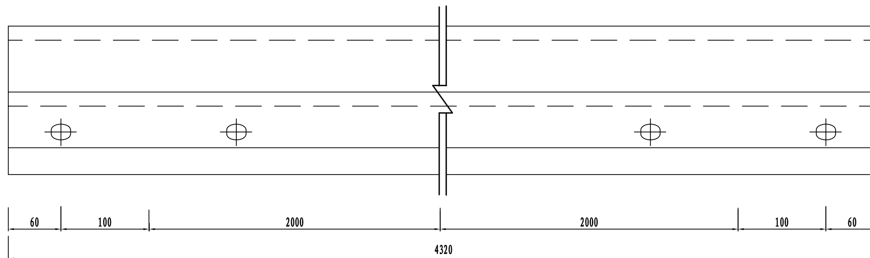
DB01' 护栏板平面图
