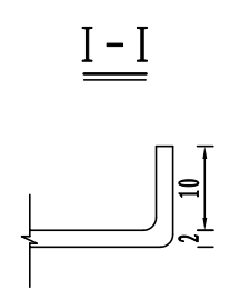
铝合金龙骨截面
