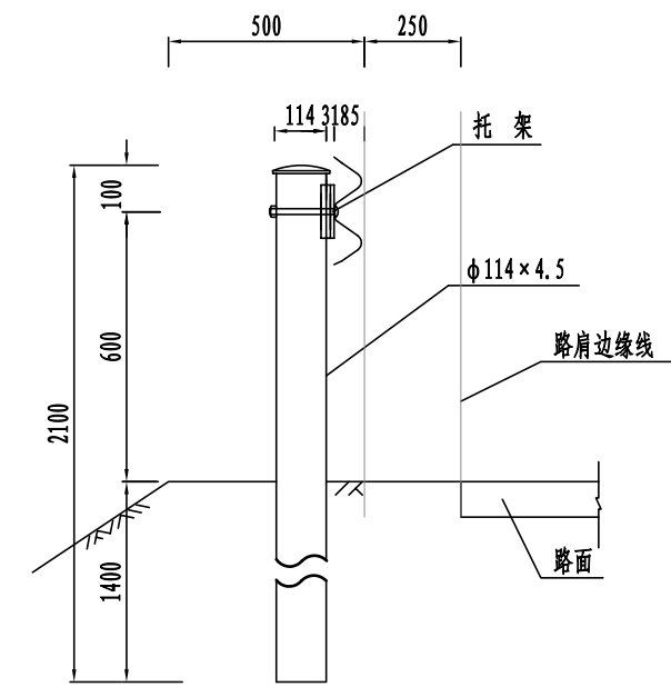
Gr-C-4E侧面图
