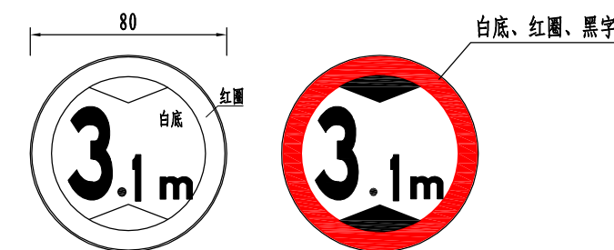
限制高度标志
