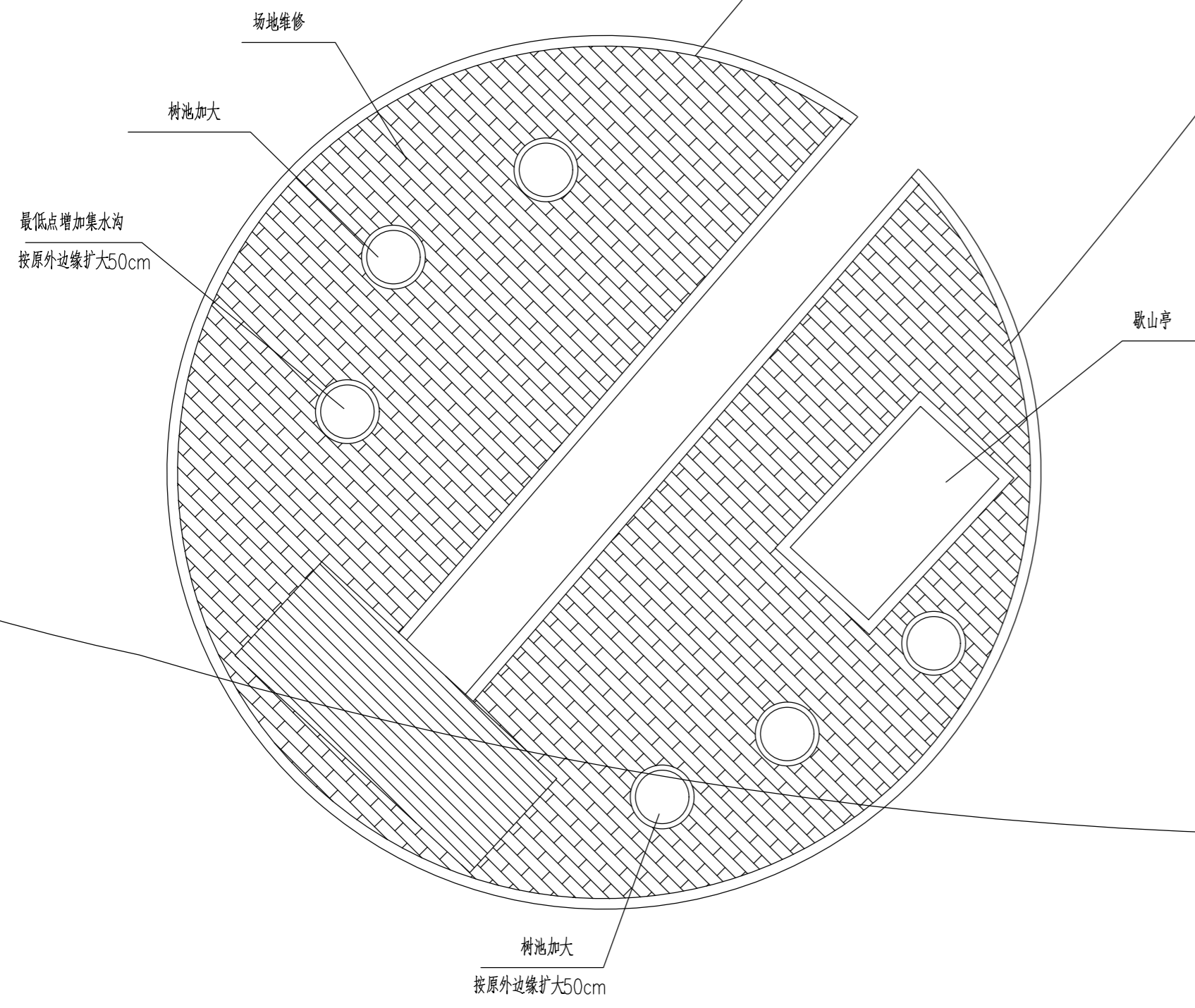
广场及亭子平面图 1:50
