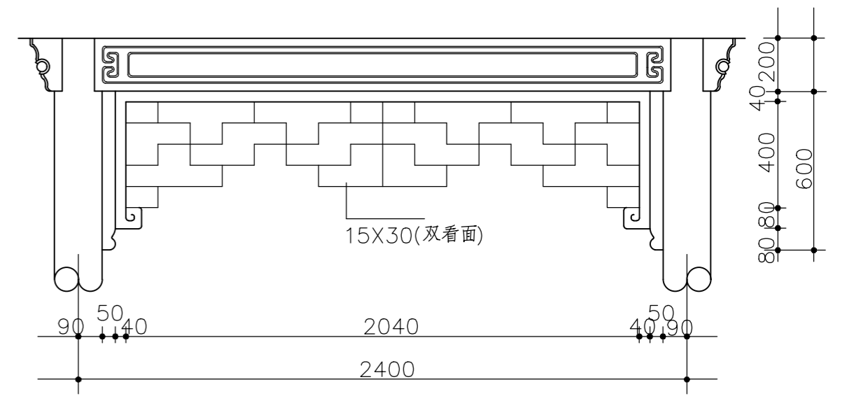
钱角大样 1/20
