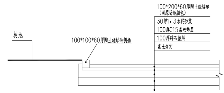
修复场地、树池剖面 1:20
