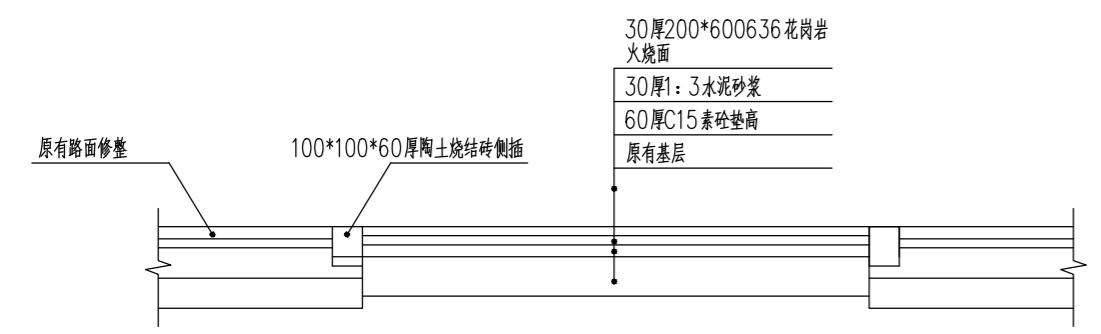
低洼路面抬高做法 1:20
