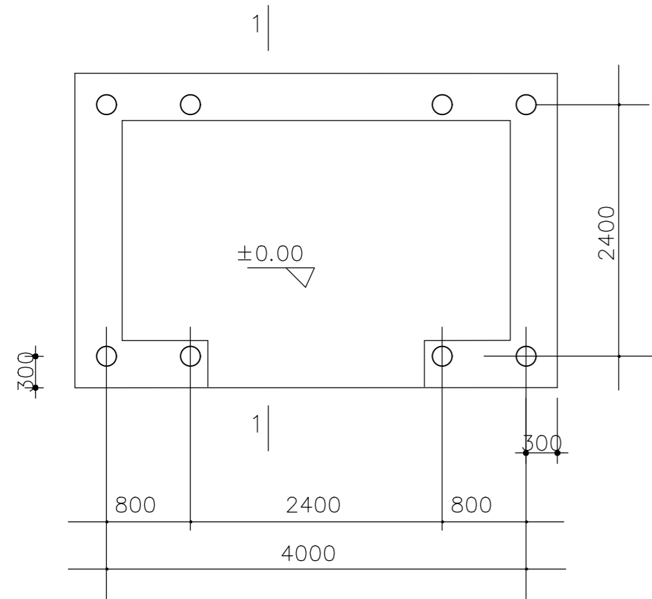
平面图 1/50
