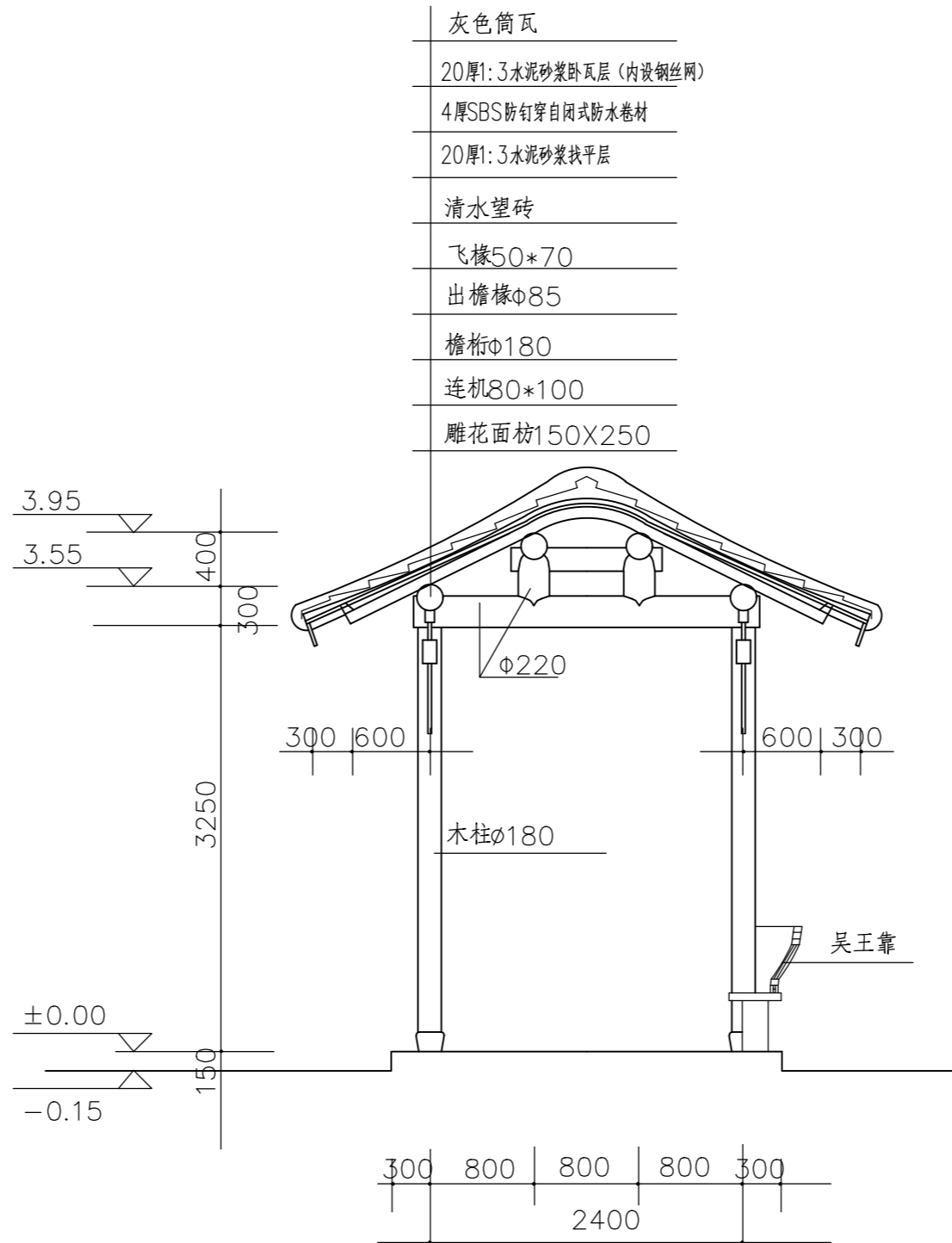
1-1剖面 1/50
