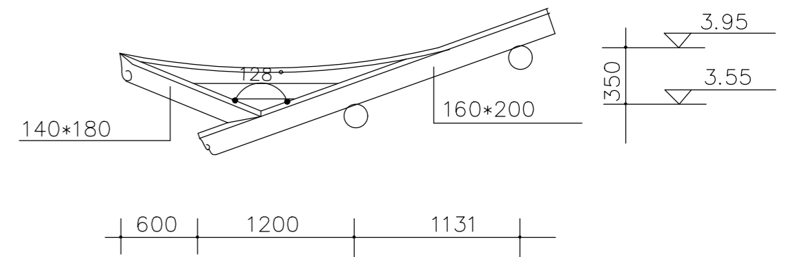
钱角大样 1/20
