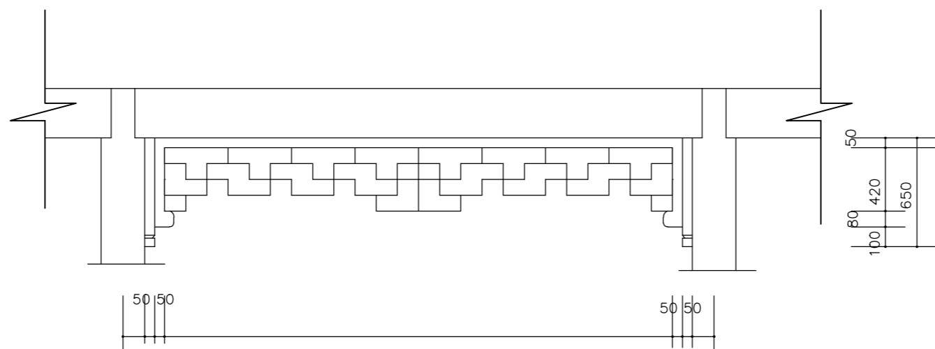
挂落示意
