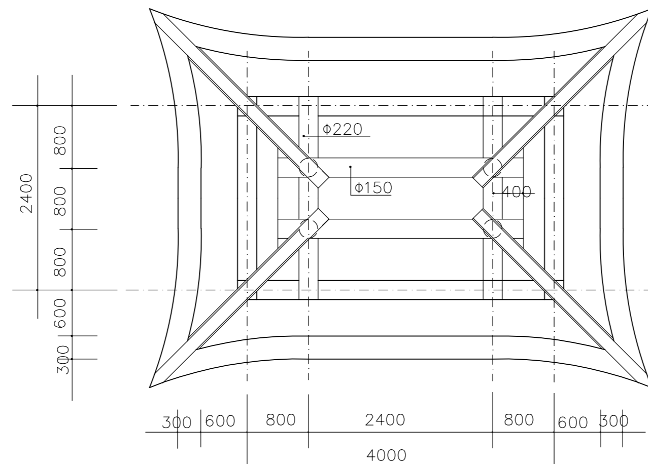
屋架平面图 1/50
