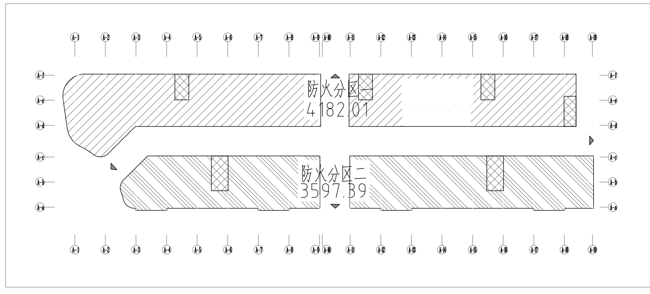
底层、二层防火分区示意图 上下层为一个防火分区
