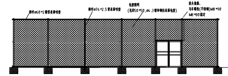
4.米高围网局立面图
