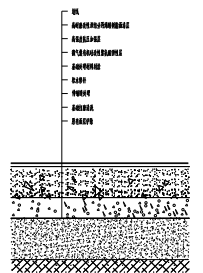
PU面层基础结构层做法 1:10
