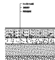
层压式EPDM面层基础结构层做法 1:10
